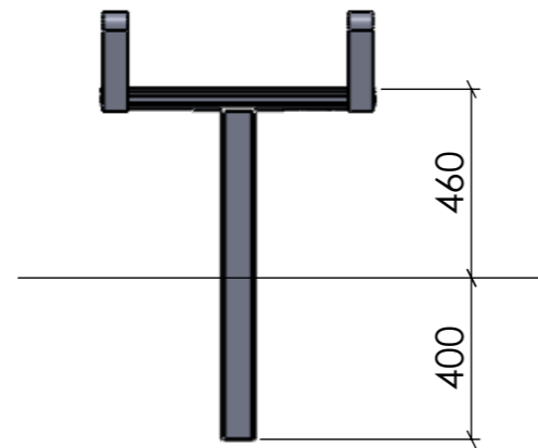
FRONTVY
