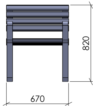
FRONTVY
