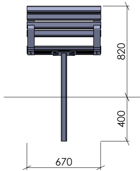
FRONTVY
