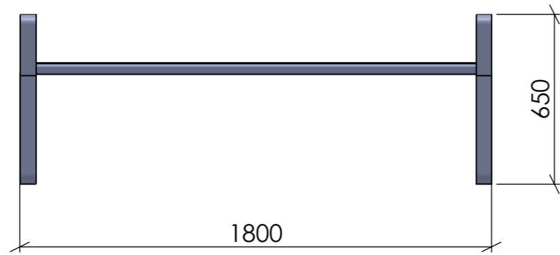
FRONTVY
