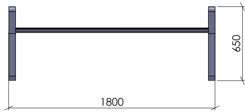
FRONTVY
