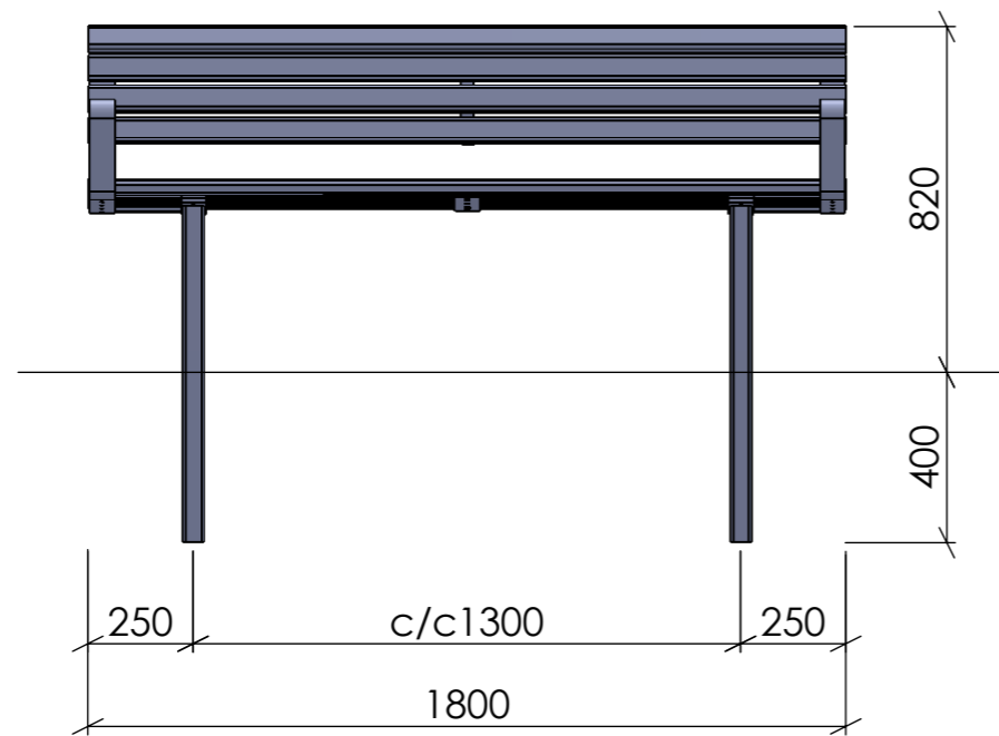
FRONTVY
